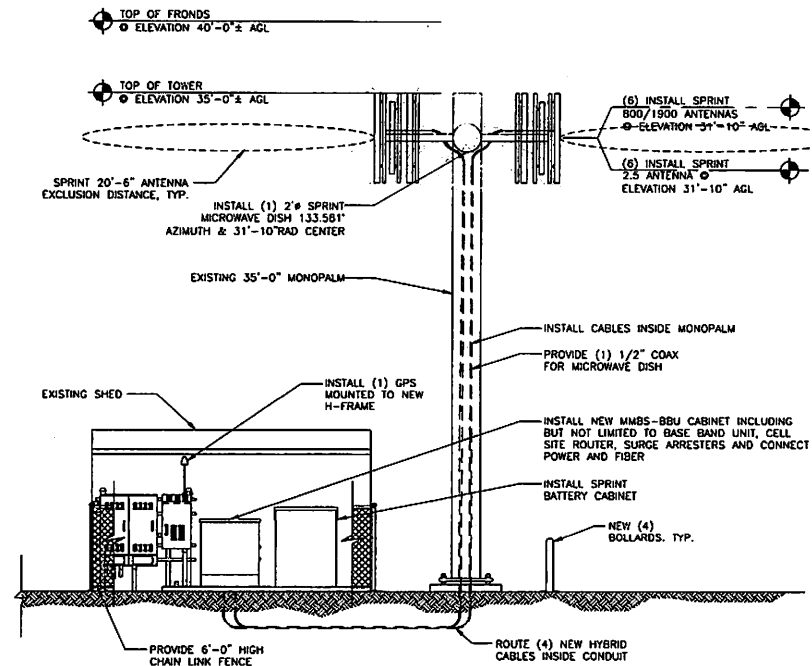
24"x38" SCALE: 1/4" = 1'-0" 11"x17" SCALE: 1/8" = 1'-0"
